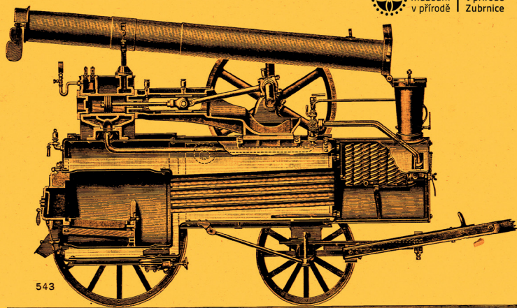
134. Parní lokomobila.
